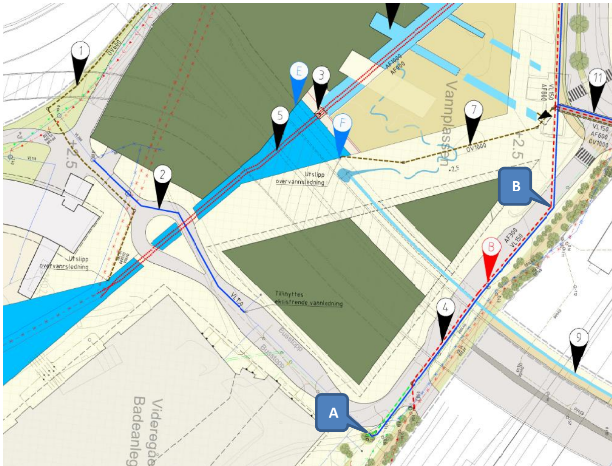
Figur 2: Utsnitt fra VA-rammeplan for Nygårdstangen. Vannledning og spillvannsledning mellom angitte punkt, A - B etableres som en del av Bybaneutbyggingen
